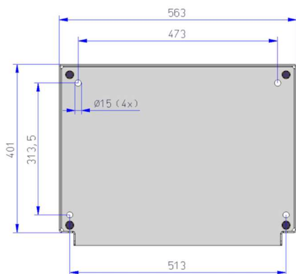
Model si dimensiuni a suportului de fixare pe trotuar / asfalt
